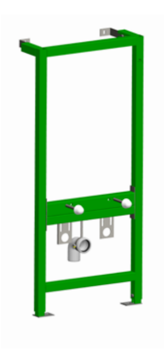
1680-010-030 VICTORIA mounting frame for bidets Застенный модуль ВИКТОРИЯ к застенной застройке биде
